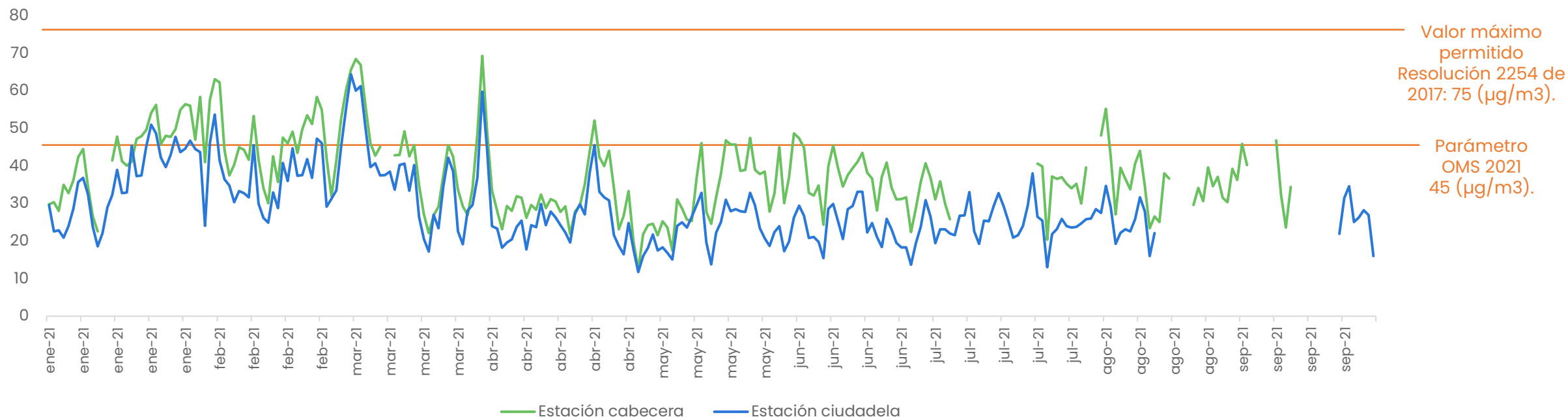
Mediciones diarias PM10 CDMB 2021
