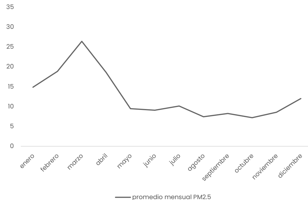
Promedio mensual PM 2,5 AMB
