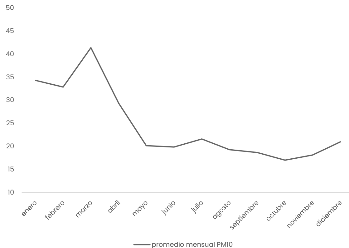
Promedio mensual PM10 AMB
