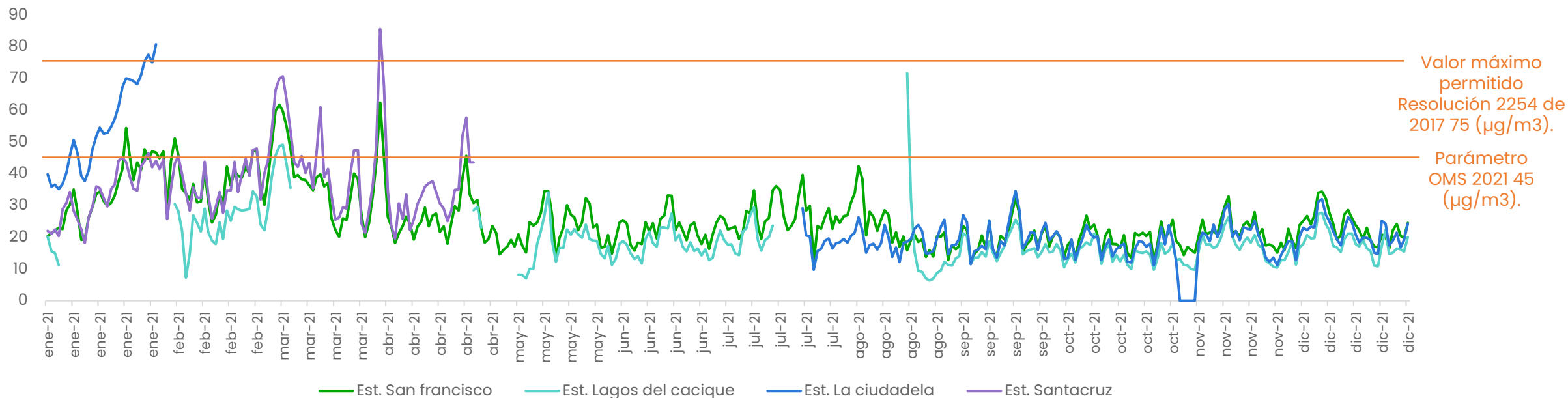
Mediciones diarias PM10 AMB 2021
