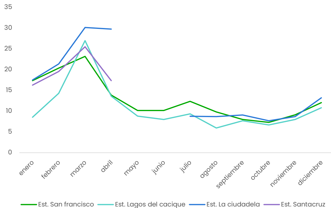
Promedio mensual PM 2,5 puntos de monitoreo AMB
