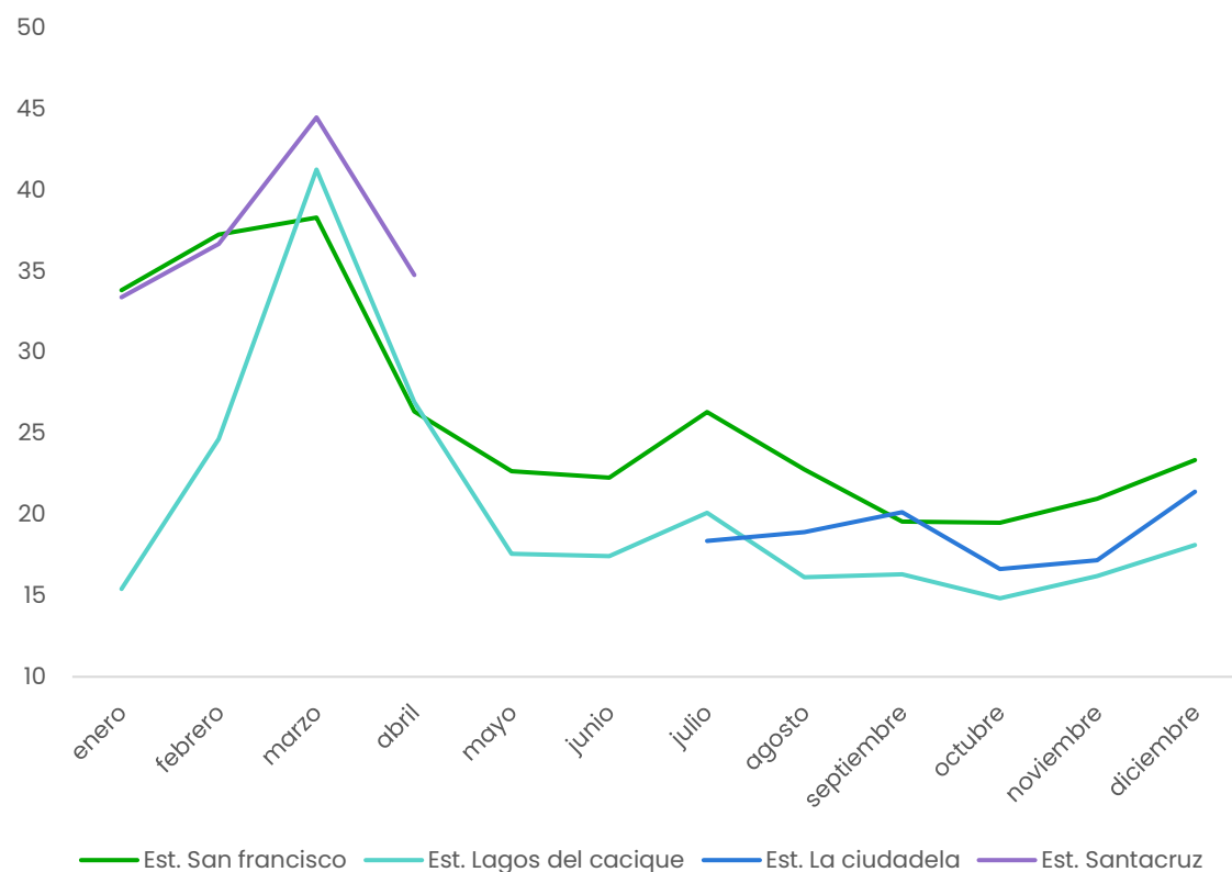
Promedio mensual PM10 puntos de monitoreo AMB
