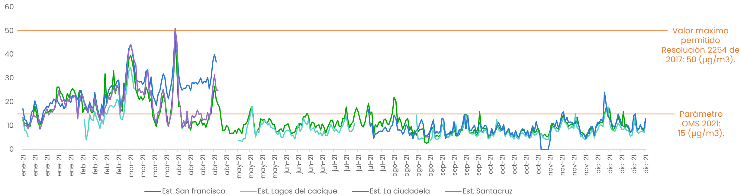
Mediciones diarias PM2,5 estaciones AMB 2021
